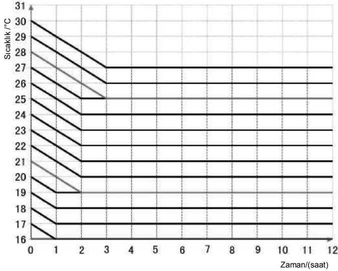
Şek.15 HEAT (ISITMA) modunda Uyku Eğrisi
